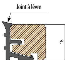
Fixclip Barre GLE18
