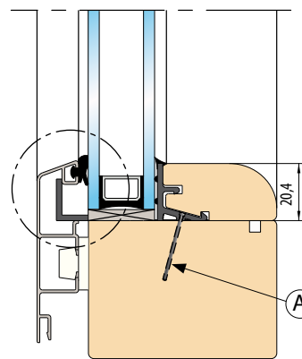
Vitrage bois-alu
