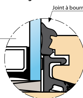
Triple vitrage IV78 FIXclip-Barre GLE 20 Plus
