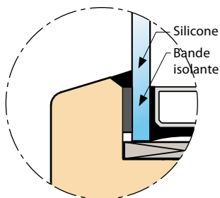
Double vitrage IV68 FIXclip-Barre GLE 18
