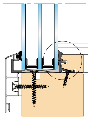
Triple vitrage fixe bois-alu IV68 FIXclip-Barre GLE 20 Plus
