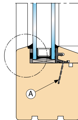
Double vitrage IV68 FIXclip-Barre GLE 18
