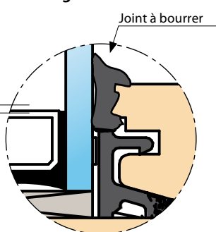
Triple vitrage fixe bois-alu IV68 FIXclip-Barre GLE 20 Plus
