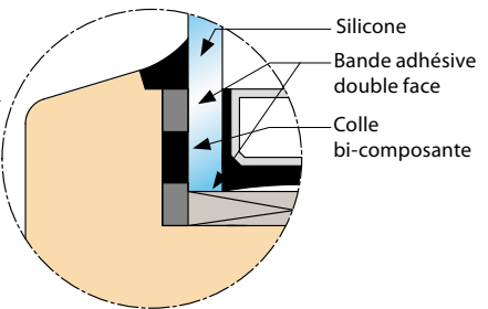
Double vitrage IV68 FIXclip-Barre GLE 18
