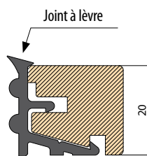
Fixclip Barre GLE20
