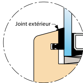
Triple vitrage IV78 FIXclip-Barre GLE 18
