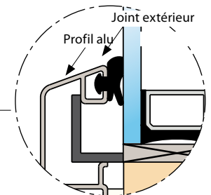
Double vitrage fixe bois-alu IV68 FIXclip-Barre GLE 20
