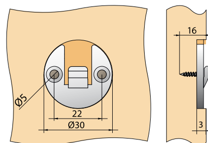
Distance d'emboîtement de 15 mm
