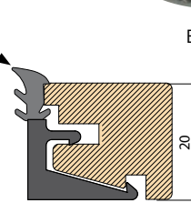
Fixclip GLE20 Plus
