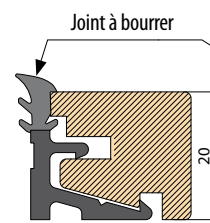
Fixclip Barre GLE20 Plus
