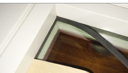
Exemple de montage : Bourrage du joint
