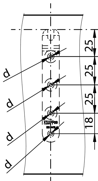
Bohrbild im Längsholz
