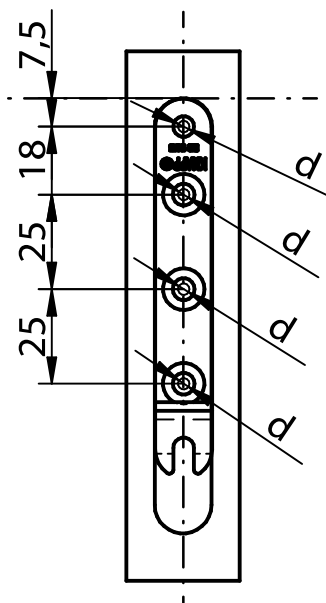
Bohrbild im Hirnholz
