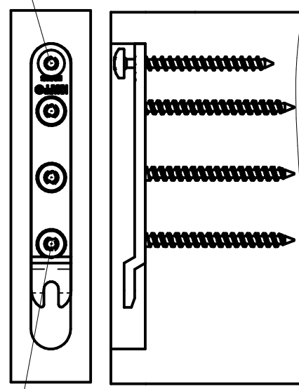
Schraubenbild im Hirnholz
