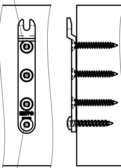
Schraubenbild im Längsholz
