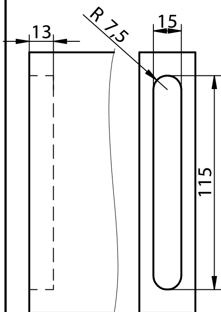
Fräsbild
