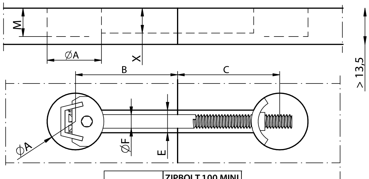
ZIPBOLT 100 MINI (Z355)
