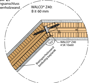
Detail B: Brettsperrholz- Außenwand- Stützenanschluss
