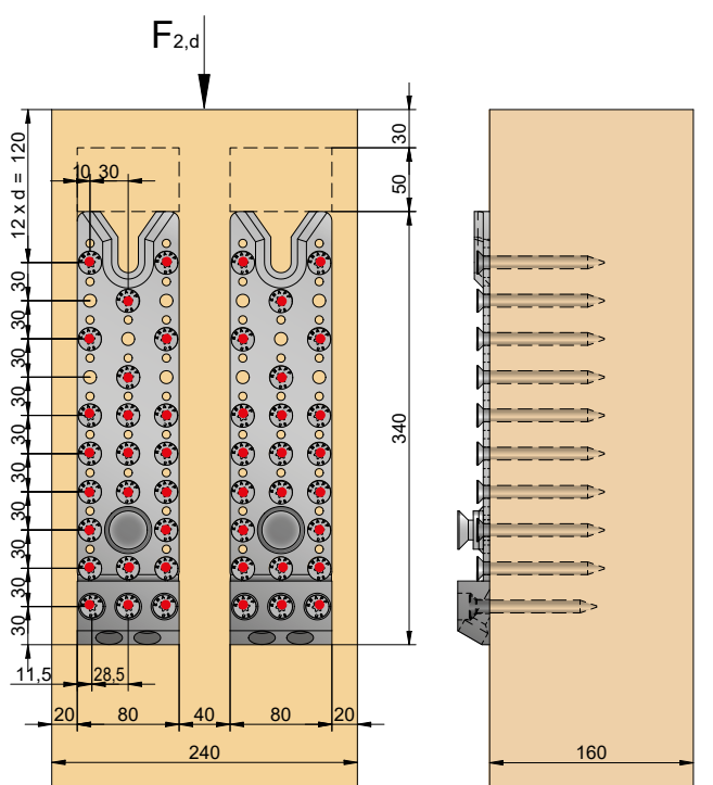
MIN. Verschraubung in Stütze
