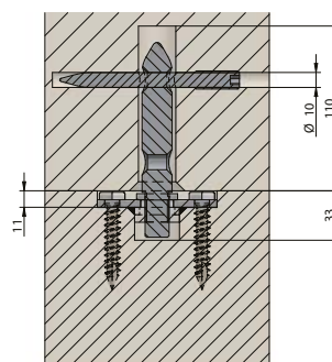
Schnitt A-A
