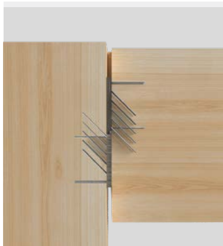
MEGANT®S – Nicht belastet
