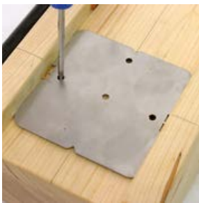
Falls erforderlich Ausfräsung herstellen, Bohrungen anzeichnen.
