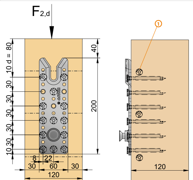
ST. Verschraubung in Stütze
