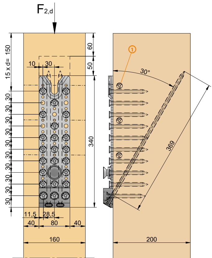
ST. Verschraubung in Stütze
