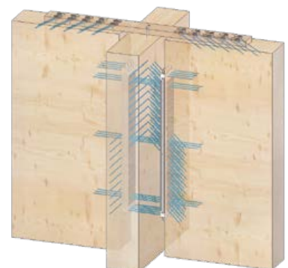
MEGANT® Haupt-Nebenträgeranschluss mit T-JOINT D35 W30 aufgeschraubter Laubholz-Zuglasche.
