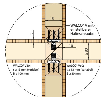
Detail F: Innenwand- Kreuzungspunkt
