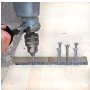
RICON®S im Hauptträger verschrauben
