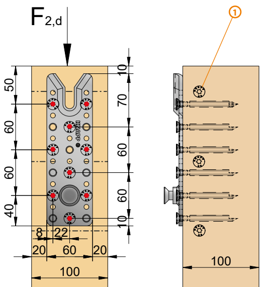
MIN. Verschraubung in Stütze
