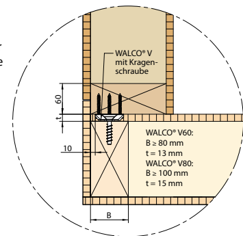
Detail A: Außenwanddecke mit durchgehender Holzwerkstoffplatte
