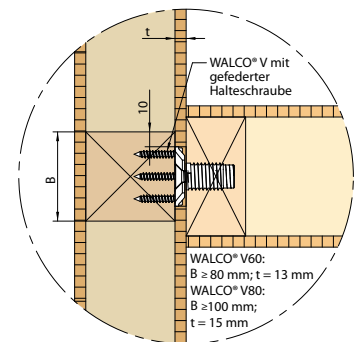
Detail D: Innenwand- Anschluss (z. B. Installationswand)
