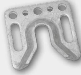
WALCO® V80 Langloch (Art.-Nr. K115/B) und Alternativ WALCO® V80 (Art.-Nr. K101/Set)
