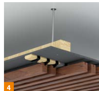
4 Leisten auf die Klammer aufstecken. Kleber abbiegen lassen.
