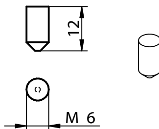
Gewindestift M6x12 ISK 3
