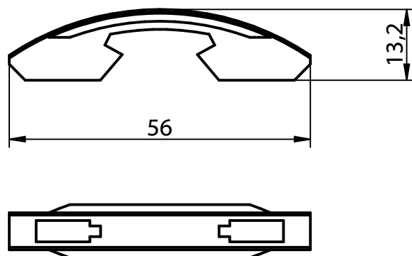
Klemmteil
