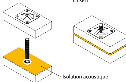
Vissage de la tige filetée dans l'insert.
