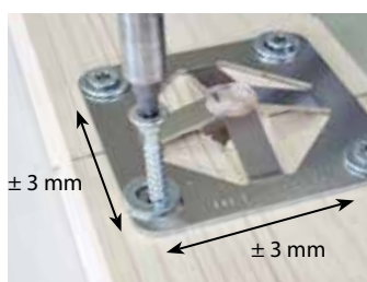
Positionnement et vissage de la platine RUKZUCK®.
