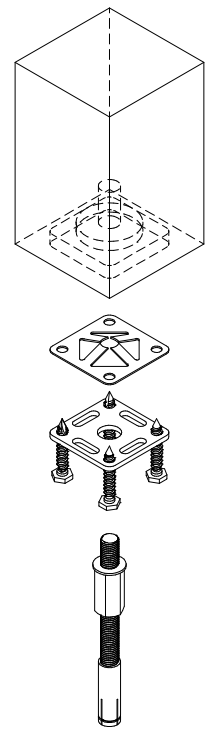
Réglage de la hauteur à l'aide de l'écrou.
