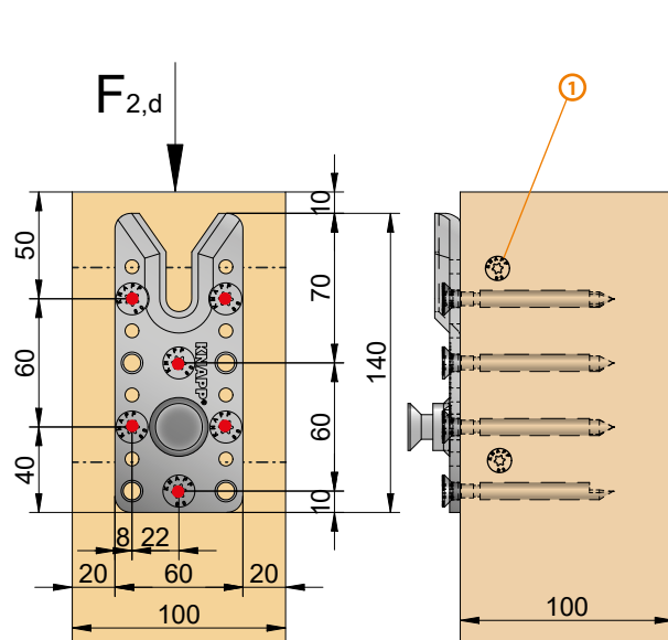
Vissage min. sur poteau
