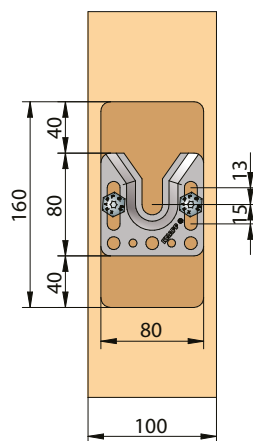
Ferrure centrée
