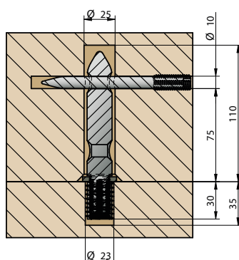
Coupe A-A
