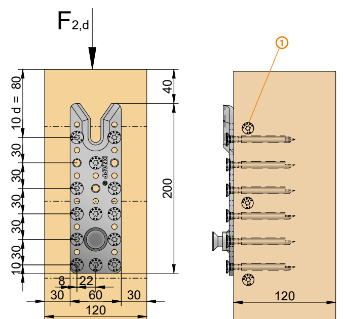
Vissage standard sur poteau
