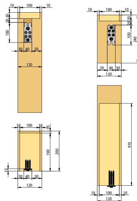
Assemblage sur panne
