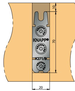
Encastrement et vissage sur poutre principale
