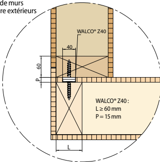
Détail B :
