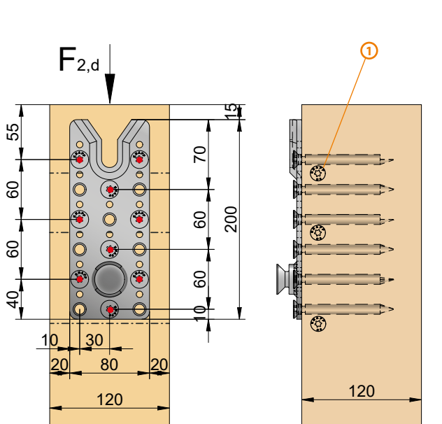
Vissage min. sur poteau
