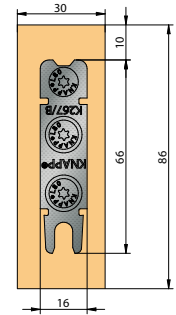
Vissage en applique sur poutre secondaire
