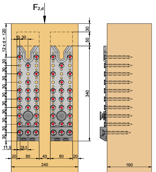
Vissage min. sur poteau
