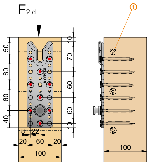
Vissage min. sur poteau
