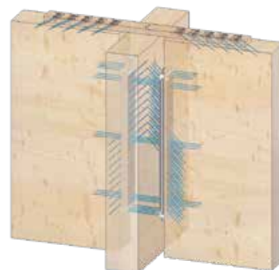
Assemblage MEGANT® de poutres principales et secondaires avec renforcement T-JOINT D35 W30 monté sur un tirant en lamellé feuillu.
