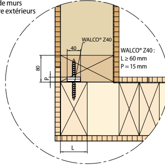
Détail C :
