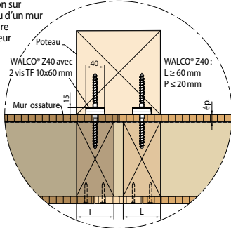
Détail D :
