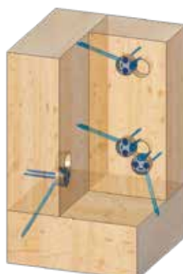
Jonction d'angles et dalle avec T-JOINT D35 W30.
