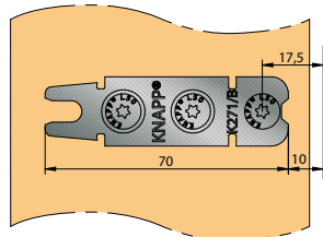
Vissage en applique sur poteau
