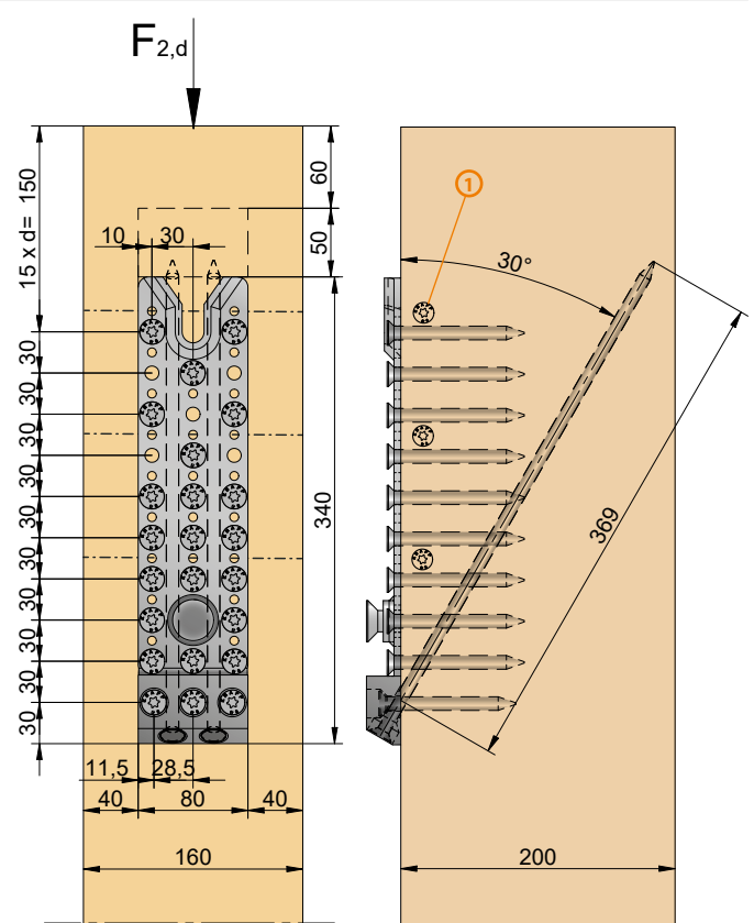
Vissage standard sur poteau
