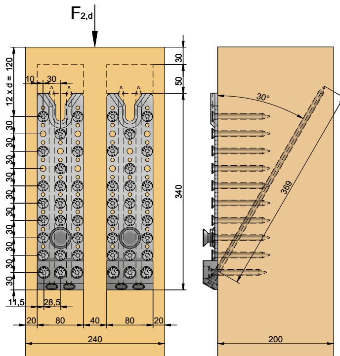
Vissage standard sur poteau
