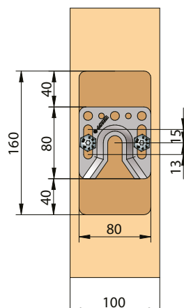
Ferrure centrée avec fourche vers le bas
