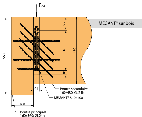
Montage encastré sur 3 côtés avec usinage en bout de panne et fixation de la plaque principale en applique sur le porteur.
