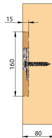
Dimensions d'usinage
