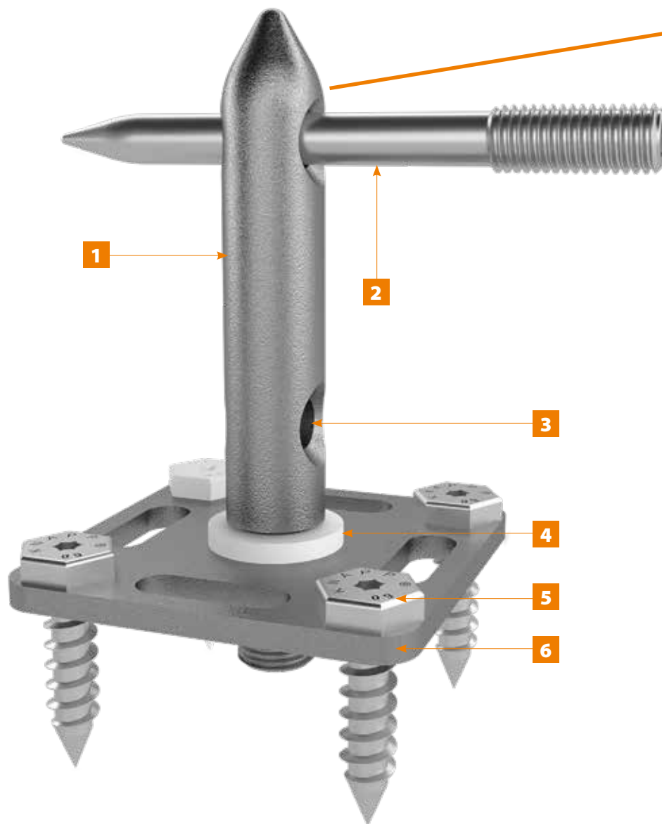
Exemple : Jonction mur-mur avec WALCO BOLT B130
