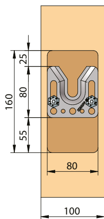
Ferrure en haut
