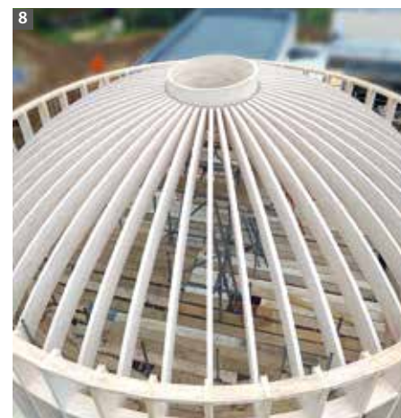
Jonctions de faitage, chevrons-poutres principales, rigides à la flexion avec T-Joint D40/W30.
