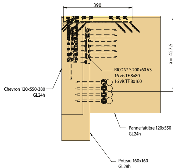
Assemblage rigide sur poteau-poutre
