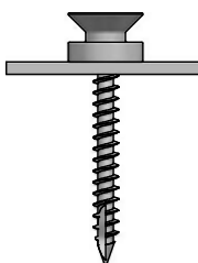
Accroche à visser (VK)
