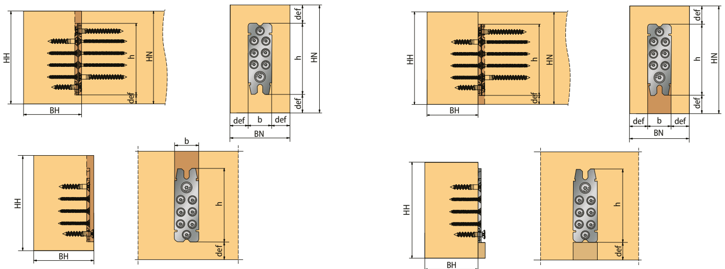
Recouvrement sur 3 côtés, encastrement sur la poutre principale
