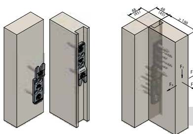
Jonction d'angle
