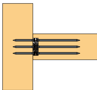
Encastrement sur la poutre secondaire
