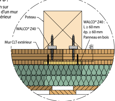
Détail D :
