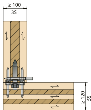
90° Visage à travers fil 90° sur CLT
