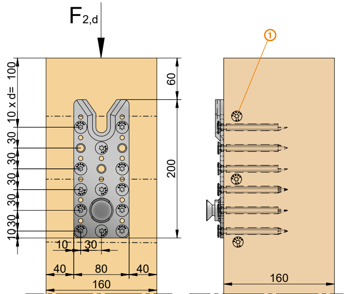
Vissage standard sur poteau
