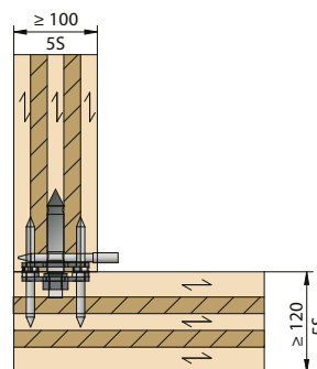
Visage par bout 0° sur CLT
