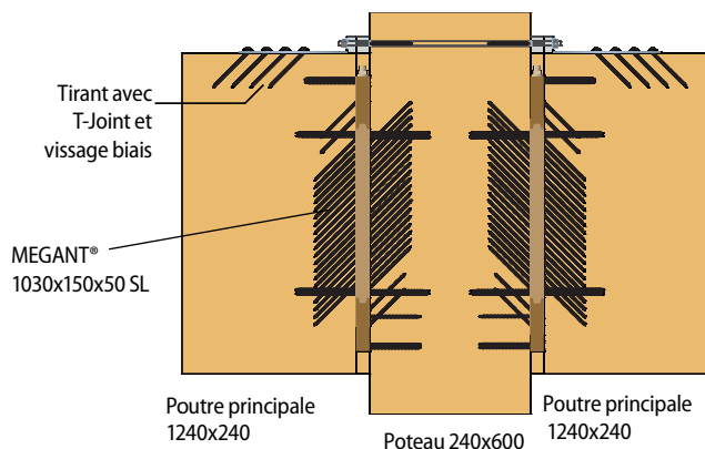
Assemblage poteau et poutres principales en face à face avec MEGANT® encastré
