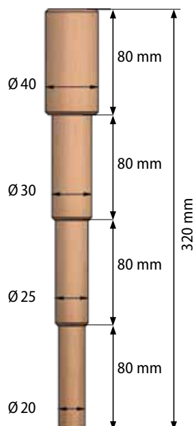
Mèche étagée
