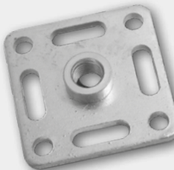
WALCO® 80 M16 avec ancrage serti (Réf. K712/B)
