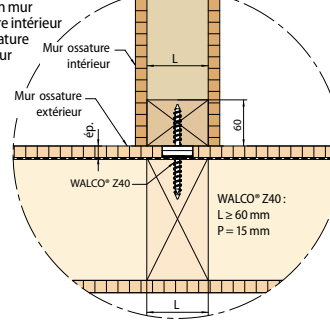
Détail E :
