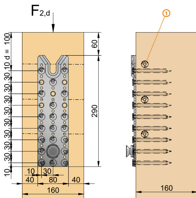
Vissage standard sur poteau
