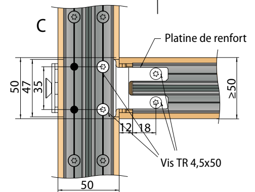
Assemblage double RICON® avec platine de renfort (VP)
