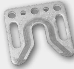
WALCO® V80 version oblong (Réf. K115/B) ou son alternative WALCO® V80 (Réf. K101/Set)
