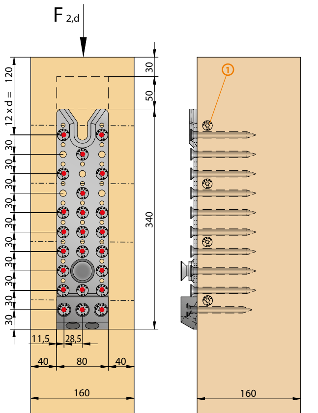
Vissage min. sur poteau
