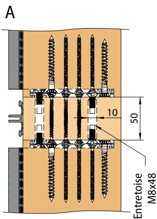
Assemblage double RICON®
