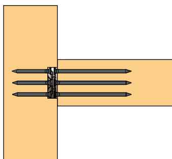
Encastrement sur la poutre principale
