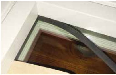
Montagebeispiel: Einbringen der Keildichtung
