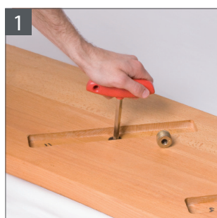
Przykręcanie nakrętki (SW10)
