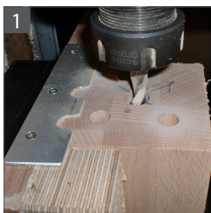
Wiercenie
