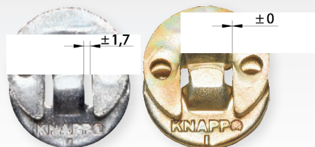
Wiercenie z szablonem
