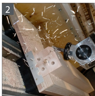
Frezowanie
