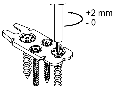
Régler la vis d'accroche
