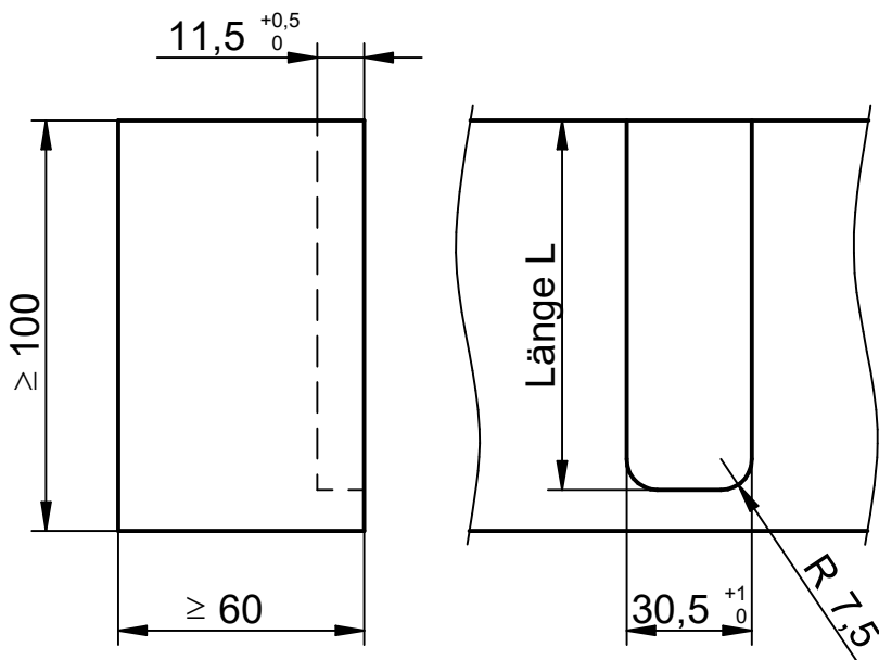
Hauptträger Fräsbild
