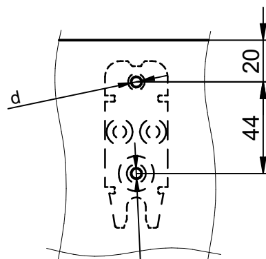
Détail du perçage sur le poteau
