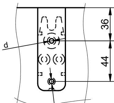
Détail du perçage sur la traverse
