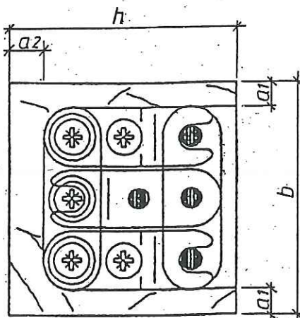
Abb. 1: Prinzipische Skizze Anschlußpunkt
