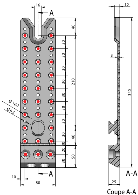
Coupe A-A
