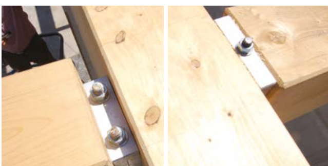
Assemblage poutres principales et secondaires en face à face avec MEGANT® en applique.
