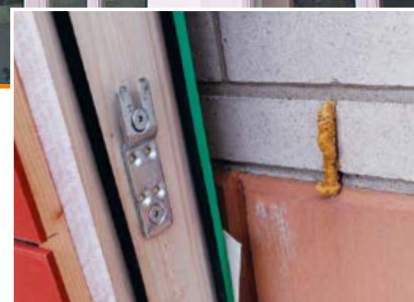
Exemple de montage : WALCO® Z40 sur montant d'ossature bois avec doubles joints
