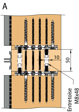
Assemblage double RICON®
