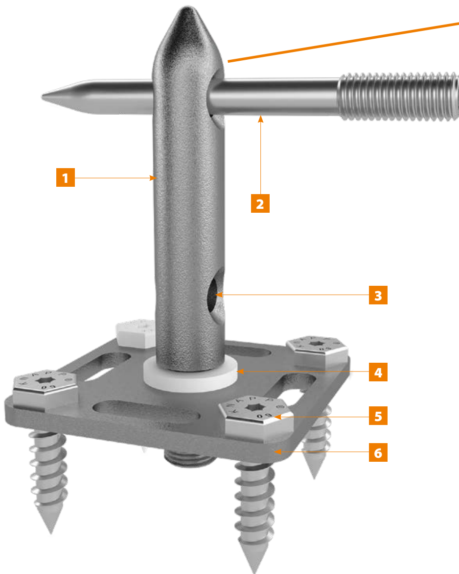
Exemple : Jonction mur-mur avec WALCO BOLT B130
