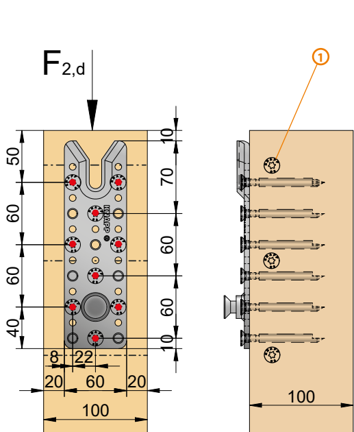
Vissage min. sur poteau
