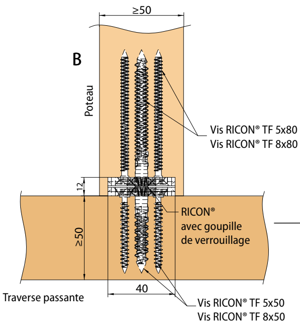
Assemblage simple RICON®
