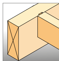
Assemblage simple : Poutre principale à partir de 100 mm Poutre secondaire à partir de 60 mm
