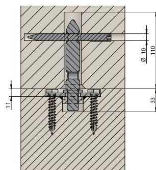
Coupe A-A
