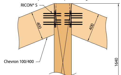
RICON®S encastré sur panne faîtière pour montage totalement invisible
