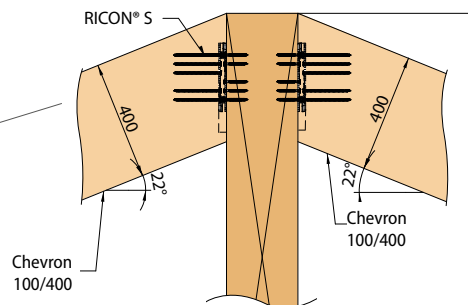
RICON®S encastré sur chevron pour montage totalement invisible
