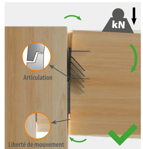
MEGANT®S – articulation de la poutre secondaire en raison de l'effort appliqué.
