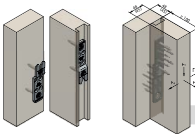
Jonction d'angle
