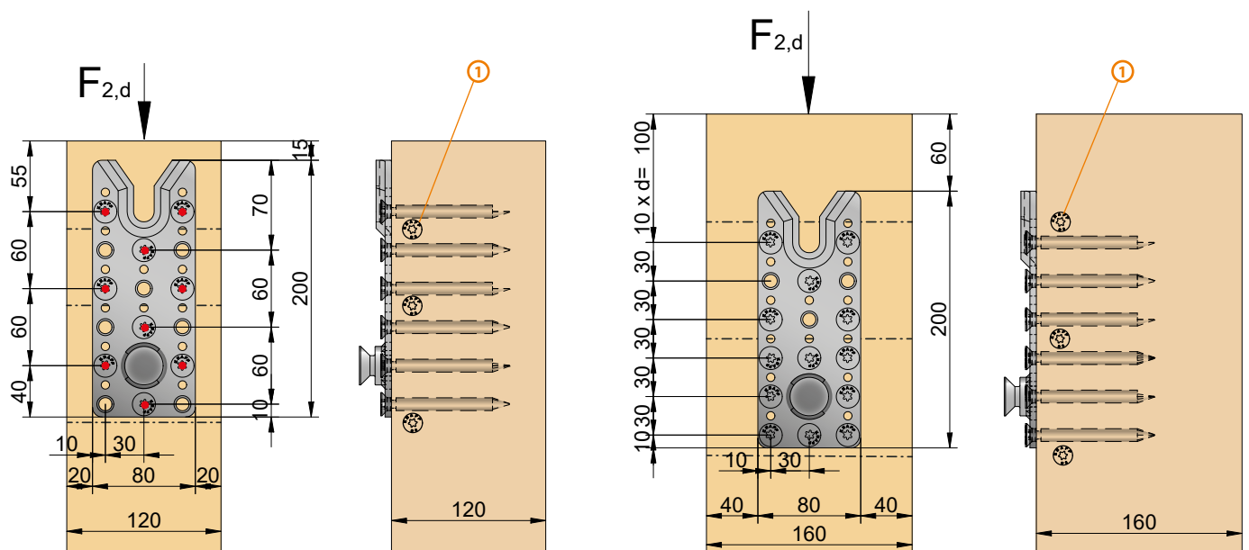
Vissage min. sur poteau
