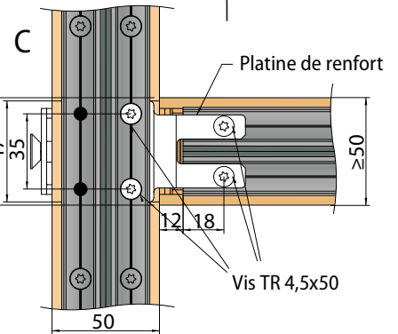
Assemblage double RICON® avec platine de renfort (VP)
