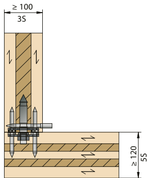
90° Vissage à travers fil sur CLT
