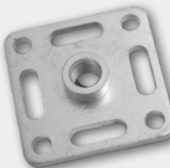
WALCO® 80 M16 avec ancrage serti (Réf. K712/B)
